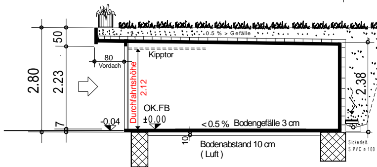
Längsschnitt
