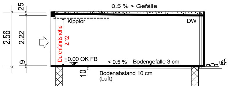
Längsschnitt
