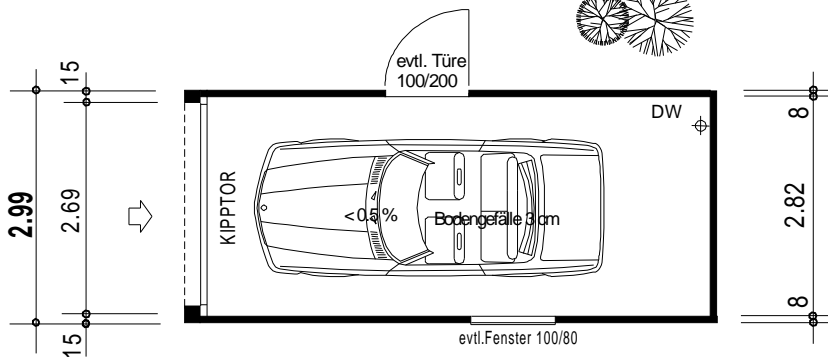
Grundriss
